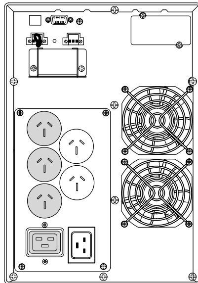
Рисунок 60. Модель PW9130G3000T-XLAU
